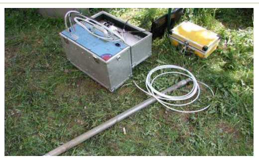
Obr. 3) CH-direkt System (direct push)
