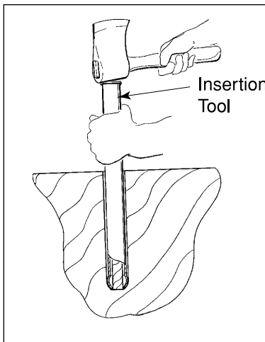
(Fig. 8a) Coring the hole
